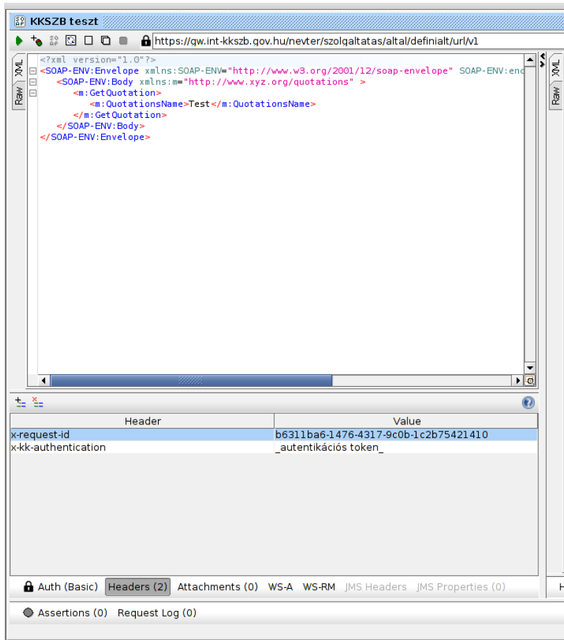
Ábra 6. SoapUI tesztprogram beállítás példa
