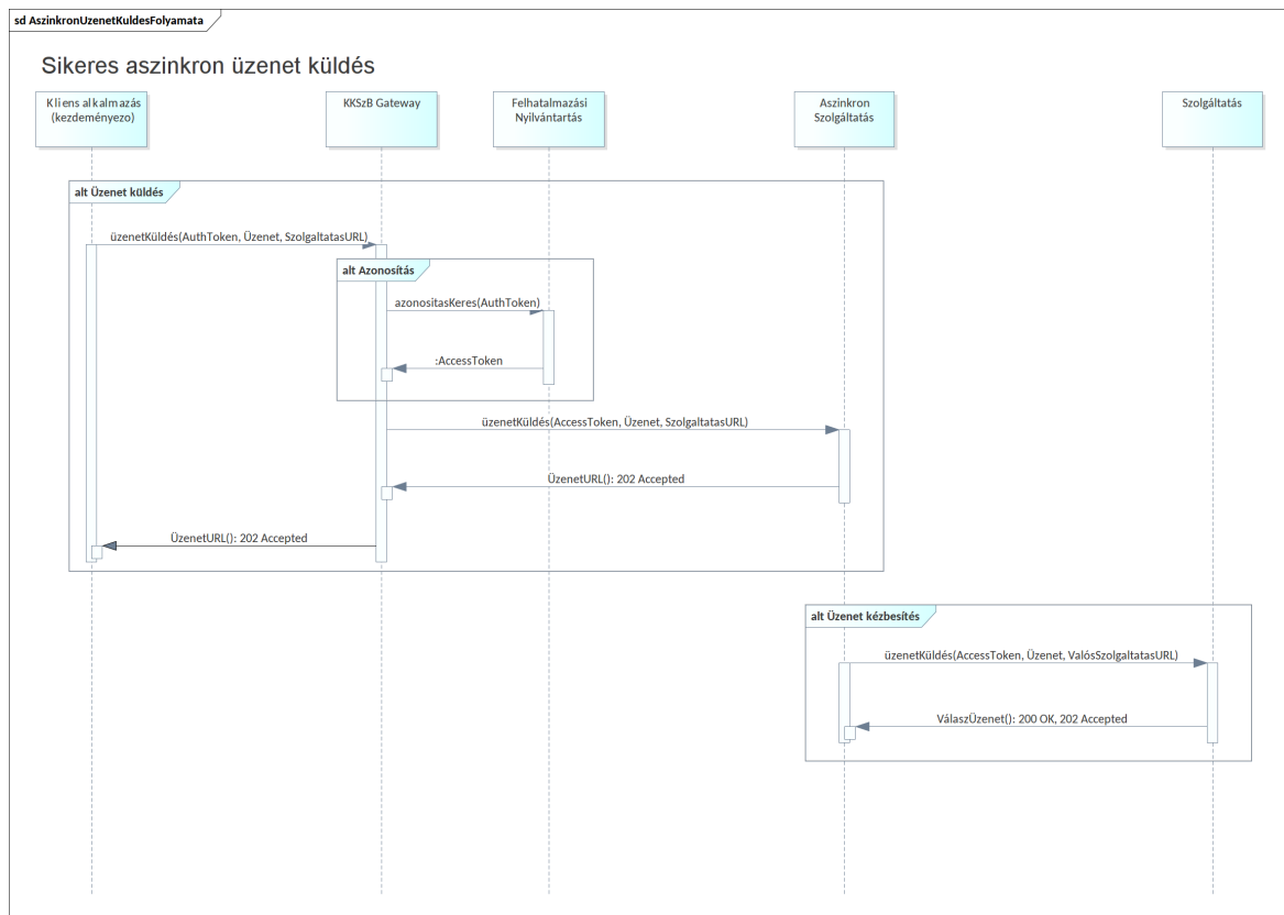
Ábra 9. KKSZB Aszinkron Szolgáltatás sikeres üzenetküldési folyamata
