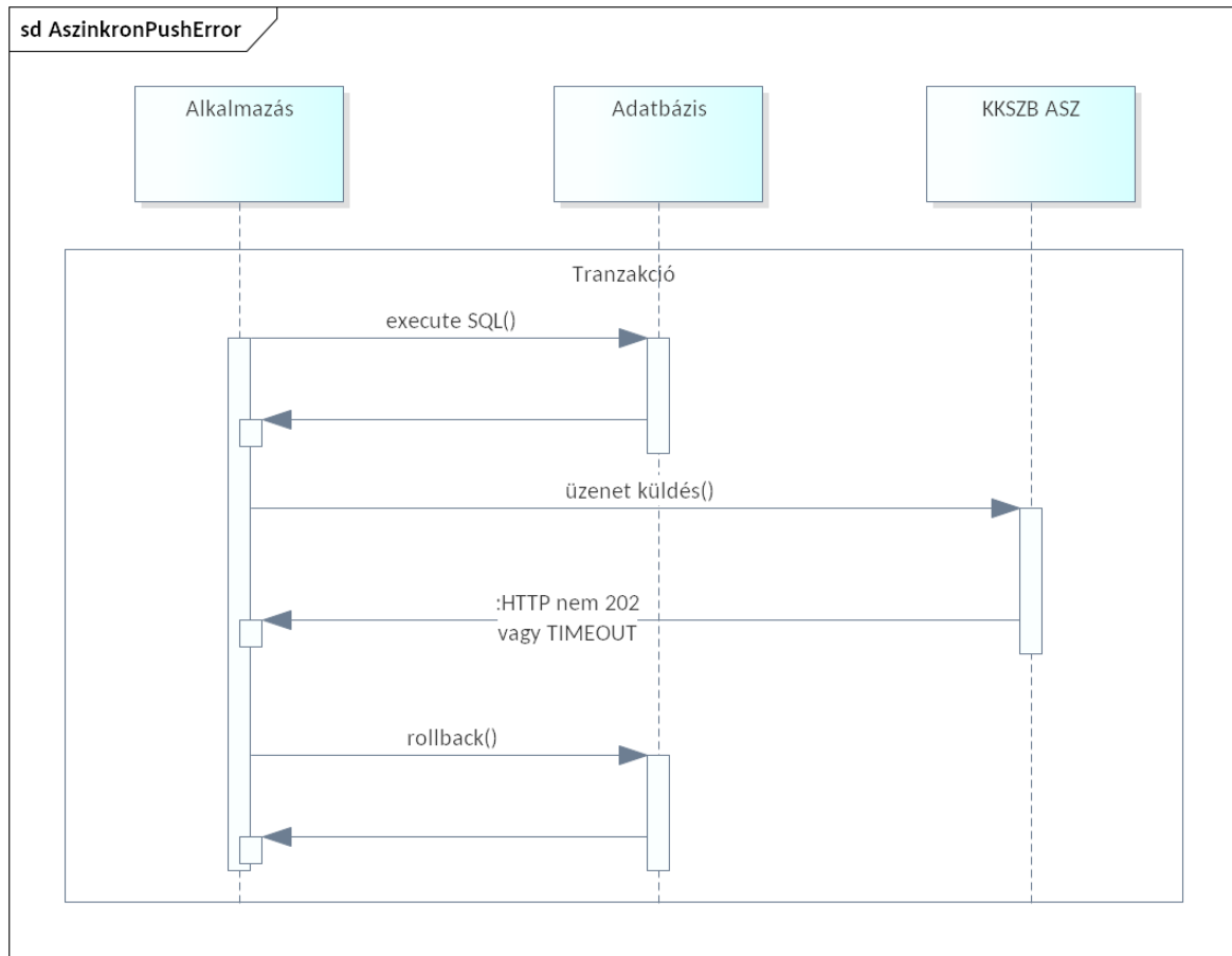
Ábra 11. KKSZB Aszinkron Szolgáltatás sikertelen üzenetküldés esetén
