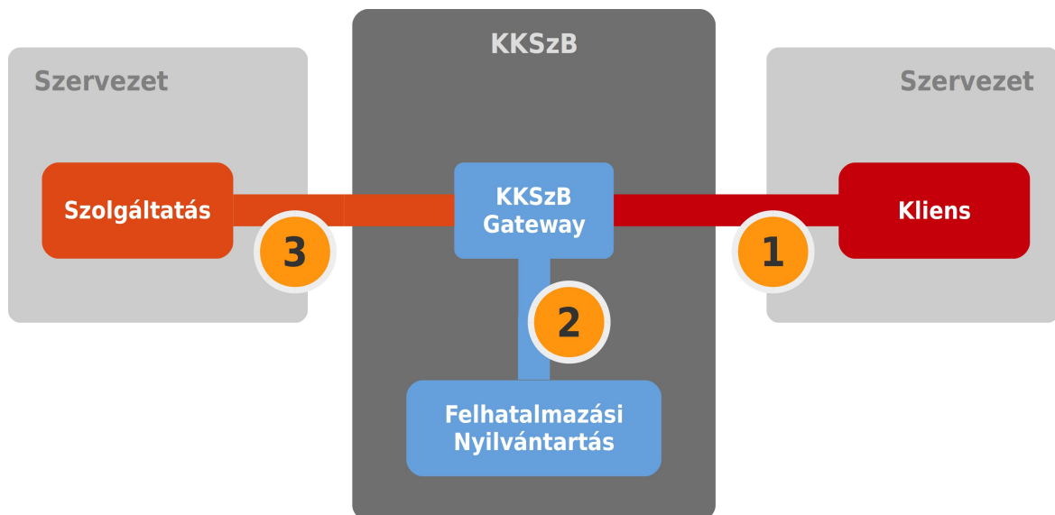
Ábra 1. KKSZB kliens alkalmazás és szolgáltatás elhelyezkedése a KKSZB rendszerben
