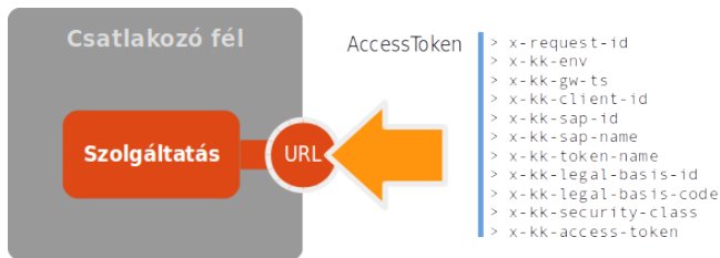
Ábra 3. Alkalmazás szintű teszt: valós szolgáltatási végponton
