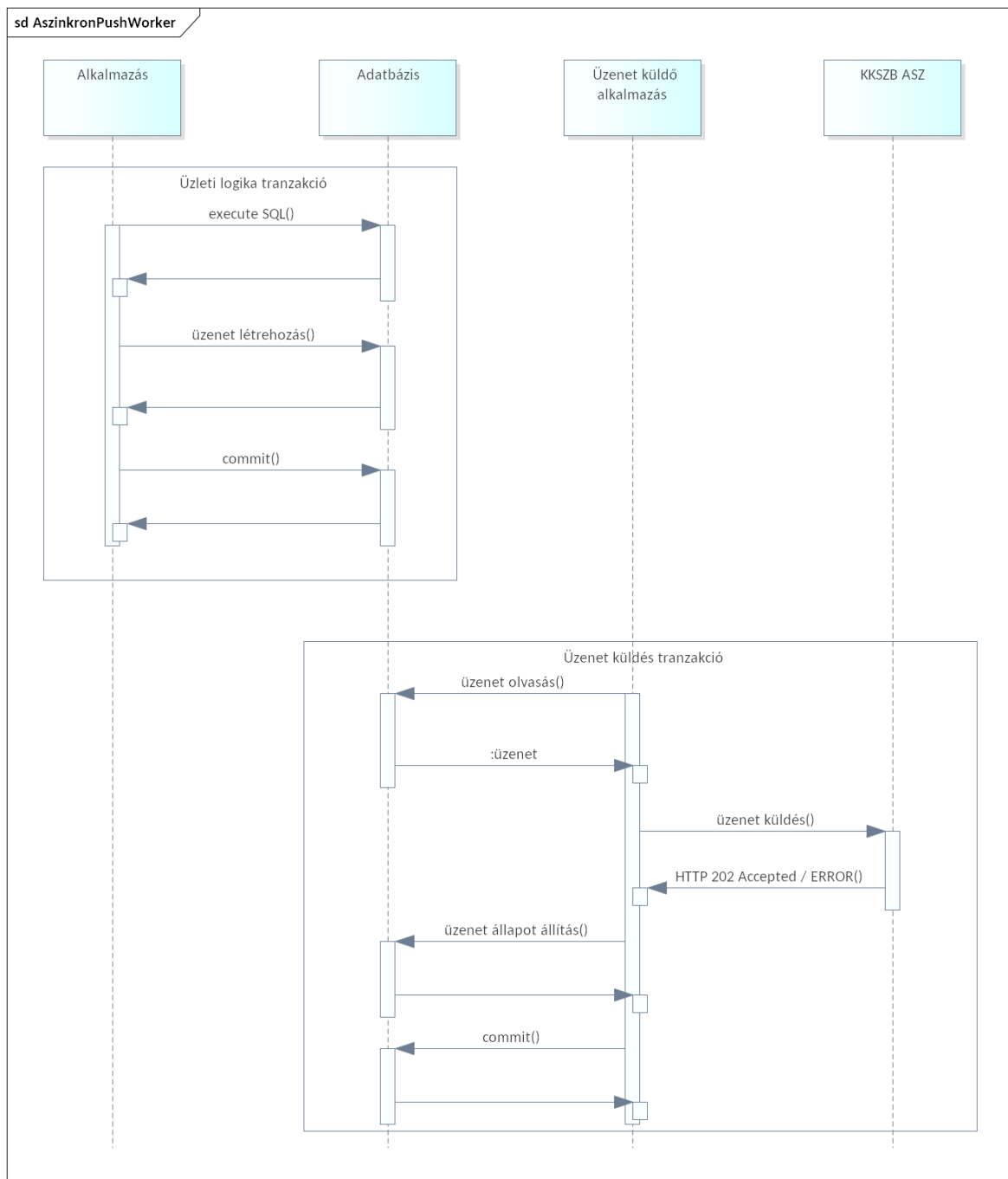
Ábra 12. KKSZB Aszinkron Szolgáltatás: nem blokkoló üzenetküldés
