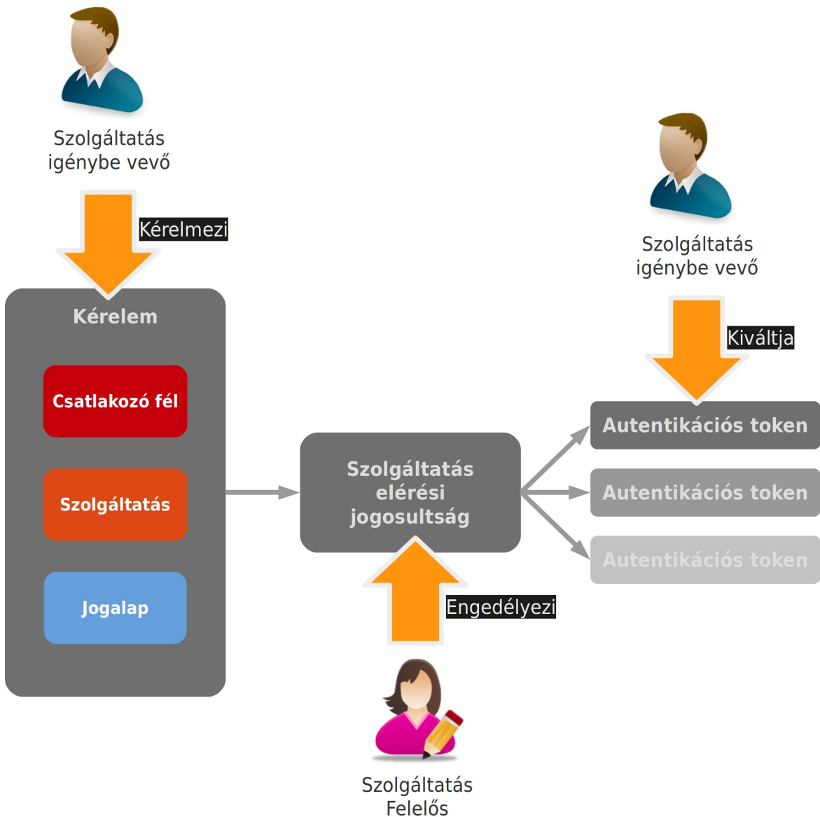
Ábra 2. Kliens autentikációs token megszerzése
