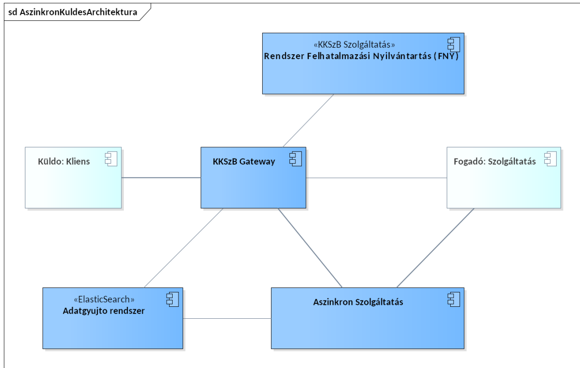
Ábra 8. KKSZB Aszinkron Szolgáltatás magas szintű architektúrája
