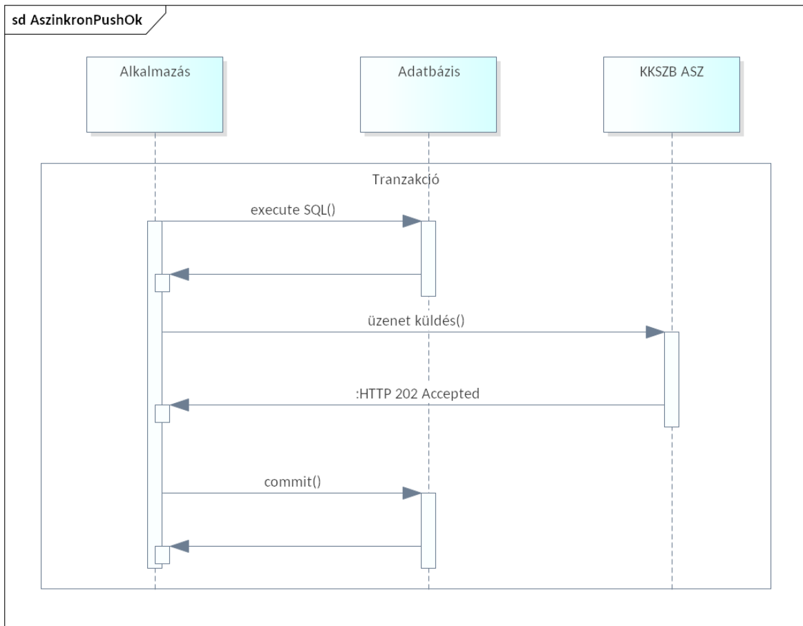
Ábra 10. KKSZB Aszinkron Szolgáltatás sikeres üzenetküldés esetén
